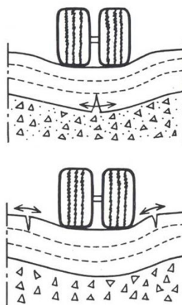
Päällysteen väsyminen
