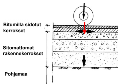
Kuormitetun tierakenteen kestävyyden kannalta kriittiset kohdat
